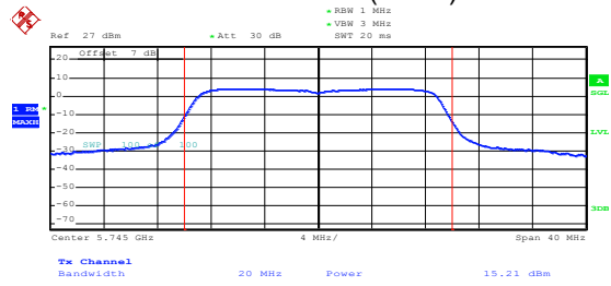
802.11ac(HT20)
