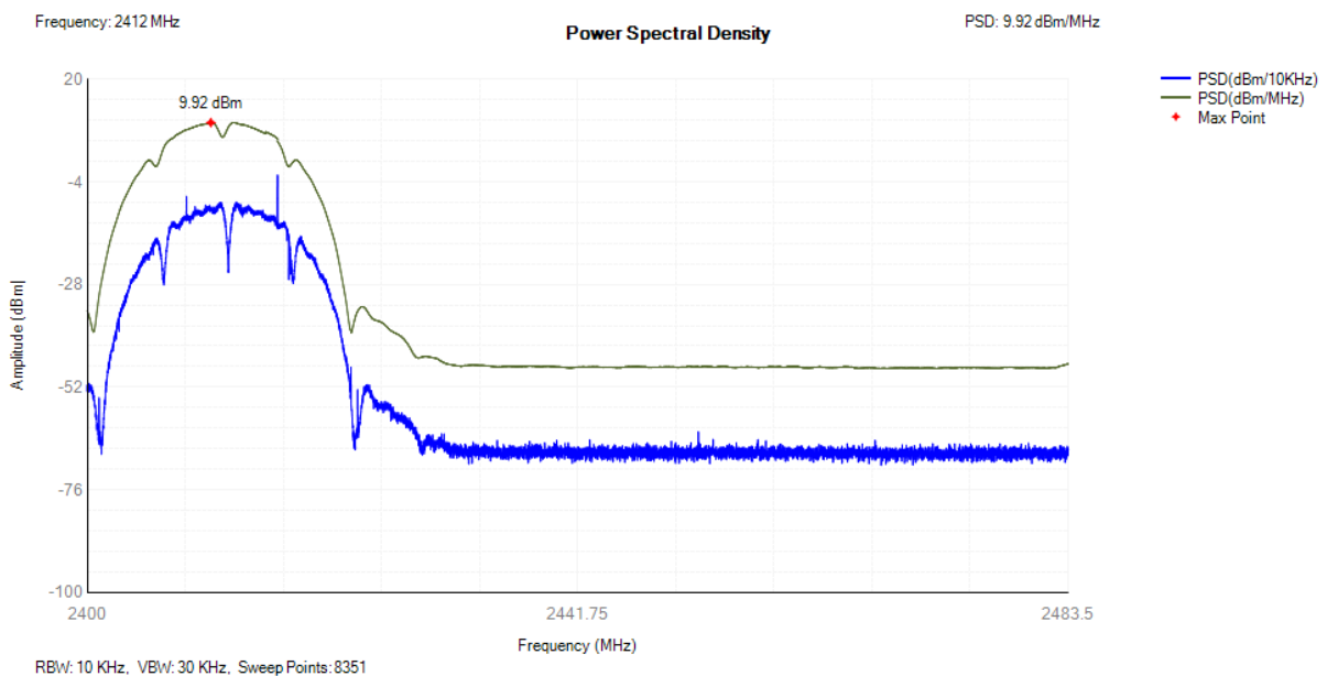
802.11b/g SISO-TX0 PSD NVNT 802.11b 2412MHz
