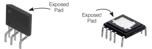
eSIP-7C (E Package)
